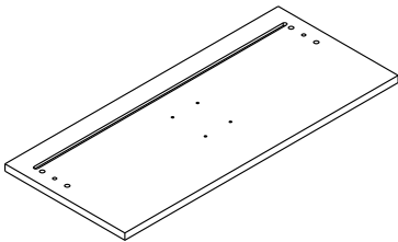
151.1.01.0009.026 x 1
